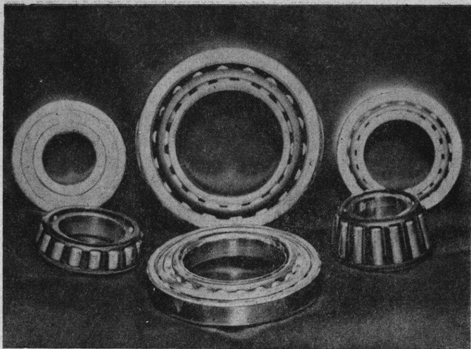
Подшипники, выпускаемые в объединении ГПЗ-4
