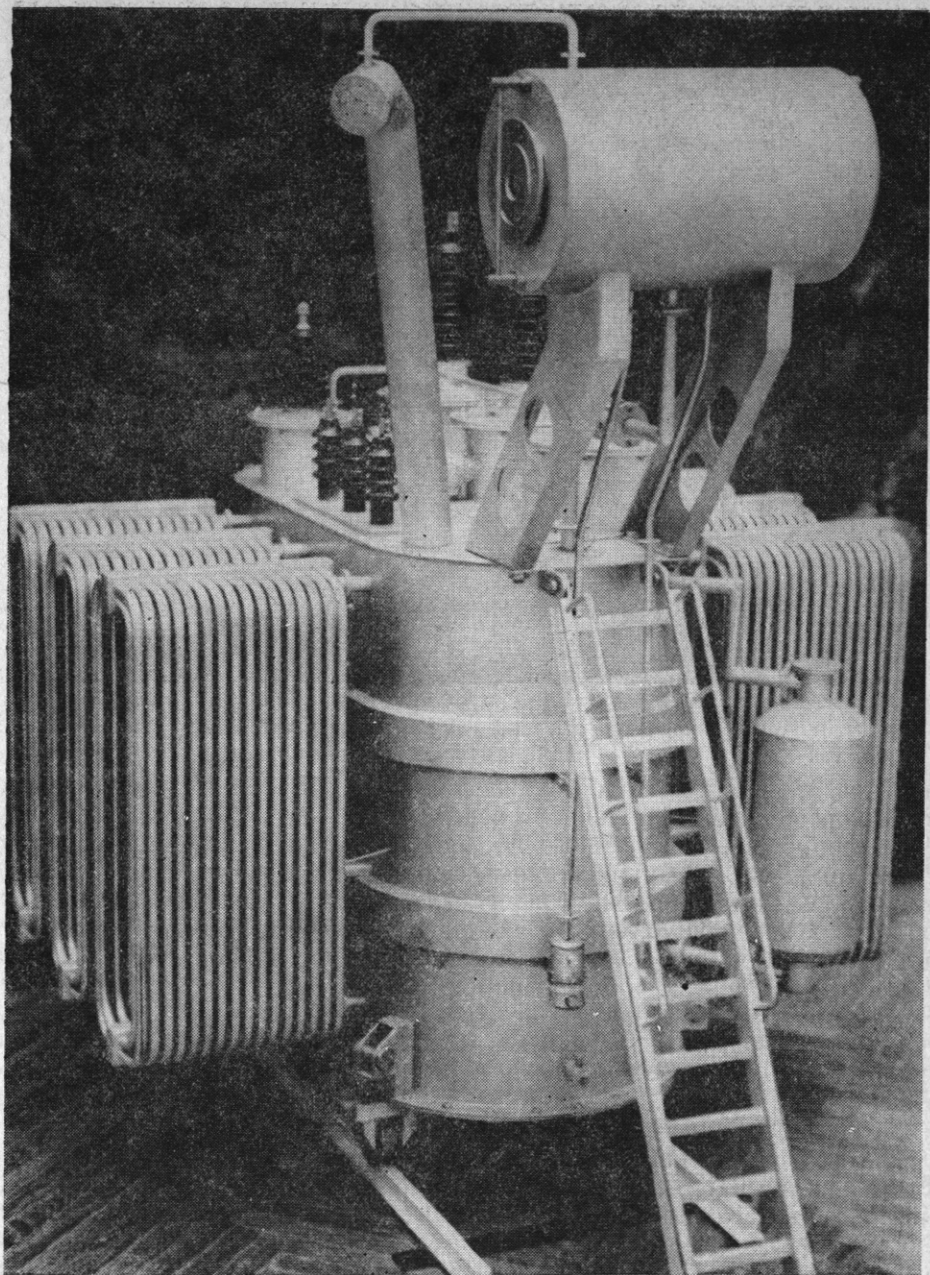
Макет трансформатора ТД-16000/66—70 (производственное объединение «Трансформатор»)
