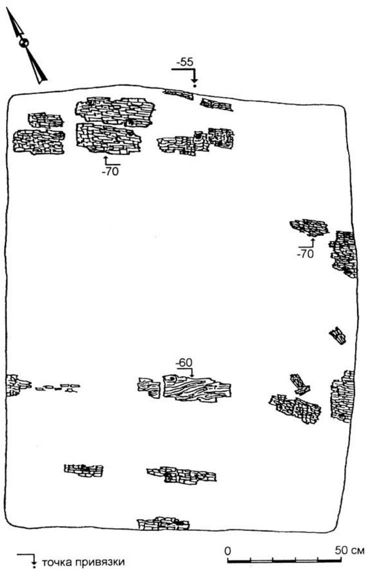
Рис. 7 Крутенький одиночный курган, погребение 4. План деревянного перекрытия.
