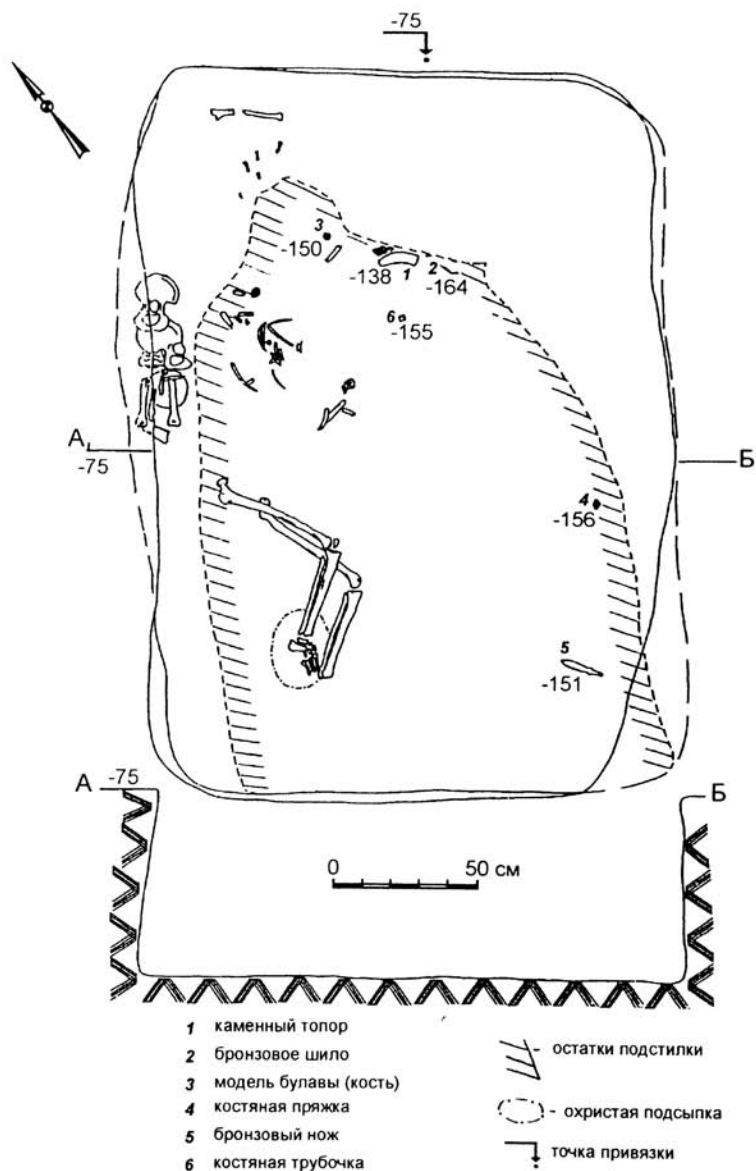
Рис.6 Крутенький одиночный курган, погребение 3.
